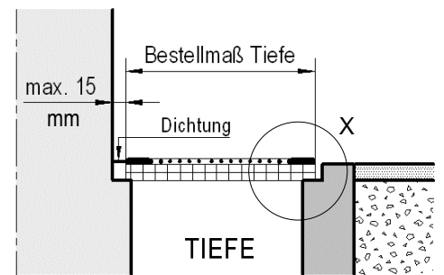
Schnittansicht Tiefe
