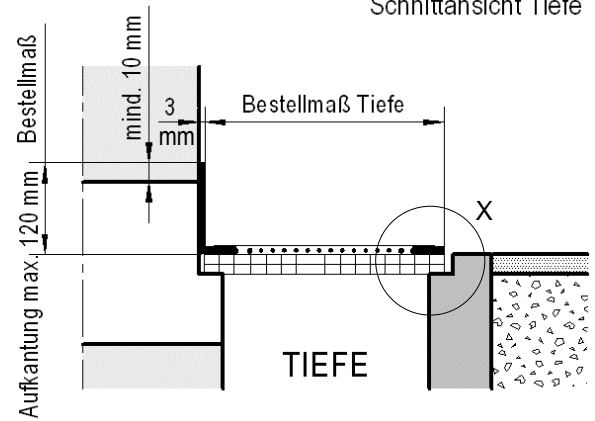
Schnittansicht Tiefe
